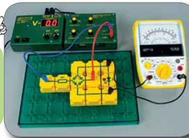
EOS 5.3.1 Můstek (proměnlivá frekvence)
